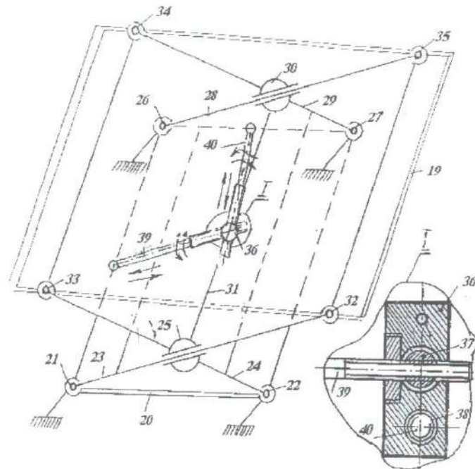
Şəkil 6. Avtomobilin yedəyini onun arxa təkərinin oxu ilə əlaqələndirən çoxbəndli oynaqlı fəza mexanizminin ümumi görünüşü (I qopartması)
