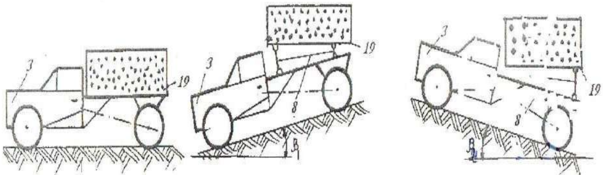
Şəkil 2. Yük avtomobili yedəyinin vəziyyətinin avtomatik tənzimlənməsi üçün intiqal mexanizminin avtomobil üzərində quraşdırıldığı vəziyyətdə yol boyu (avtomobilə yandan baxdıqda) yolun relyefindən asılı olaraq avtomobilin vəziyyətləri
