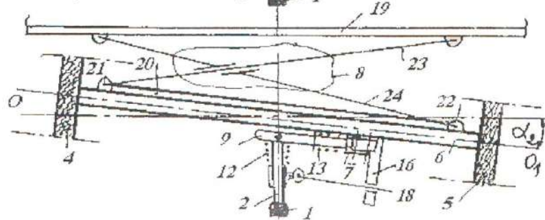
Şəkil 1. Yük avtomobili yedəyinin vəziyyətinin avtomatik tənzimlənməsi üçün intiqal mexanizminin avtomobil üzərində quraşdırıldığı vəziyyətdə yolun eni üzrə (avtomobilə arxadan baxdıqda) yolun relyefindən asılı olaraq avtomobilin vəziyyətləri
