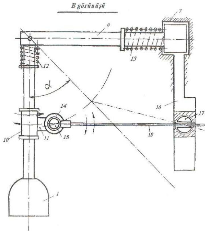
Şəkil 5. Çoxbəndli oynaqlı fəza mexanizminin kombinə edilmiş oymaqla və siqnal qurğusunun lingi ilə sərt əlaqədə olan sonsuz vint reduktorlarının ümumi görünüşü
