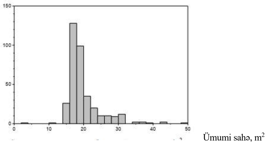
Şəkil 2. Yastı günəş kollektorlarının xüsusi kütləsinin modellərin sayına görə paylanması: a – SRCC məlumatları, b – SPF məlumatları.
