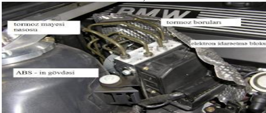
Şəkil 2a və 2b. ABS elementlərinin real görünüşü
