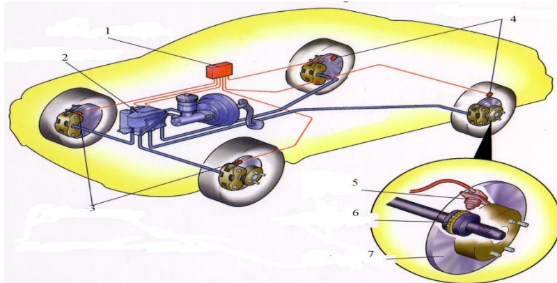
Şəkil 1. Sadə ABS - in quruluşu
