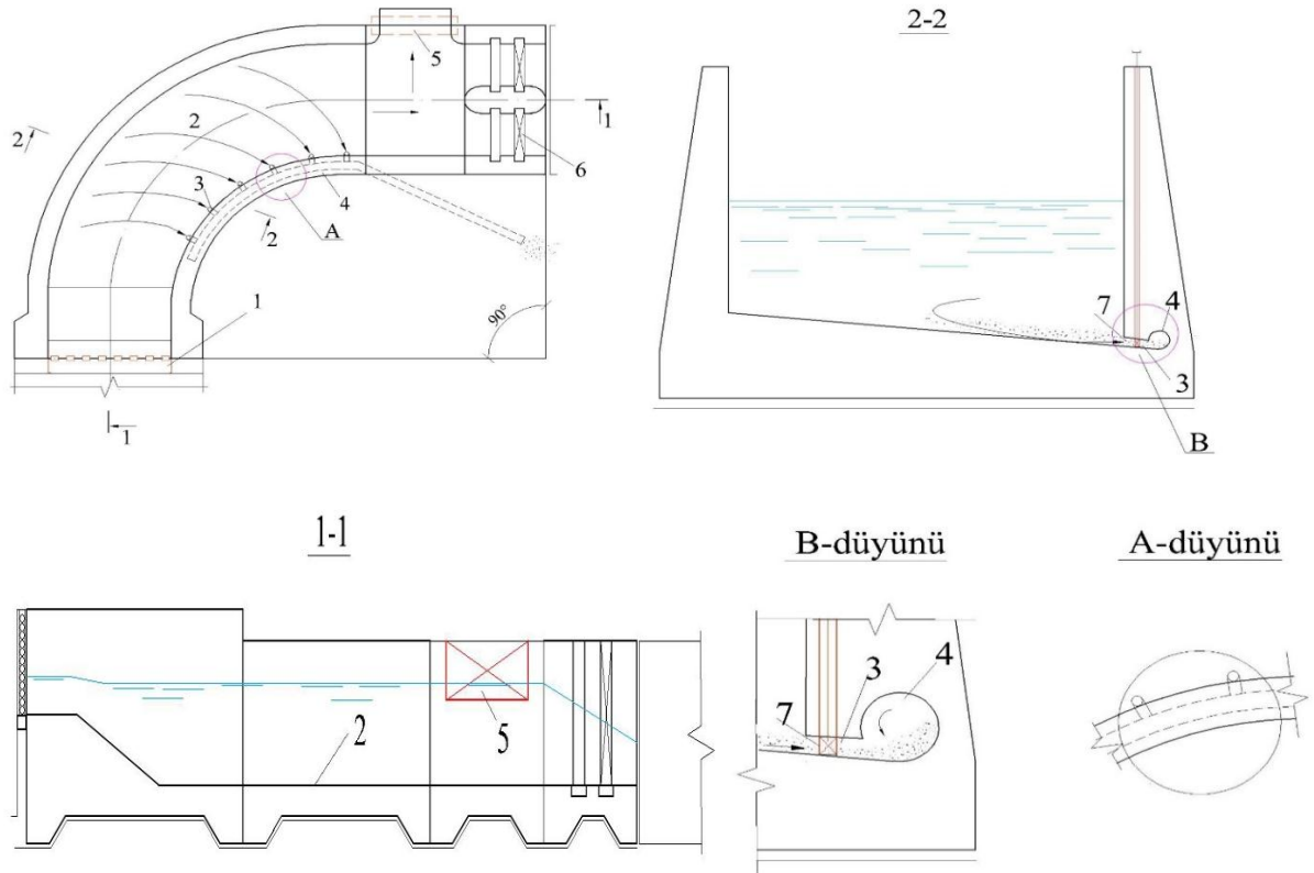
Şəkil 2. Əyrixətli durulducunun plan və kəsikləri: suqəbuledicinin metal barmaqlığı – 1; durulducu kamerası – 2; qabarıq divarının aşağısında dairəvi en kəsikli yuyucu borucuqları – 3; yığıcı element – 4; durulducunun çökük divarında suqəbuledici bağlayıcı – 5; durulducunun sonunda yuyucu bağlayıcılar – 6; Qabarıq divarın daxilində yuyucu borucuqların işini tənzimləmək üçün bağlayıcılar – 7.
