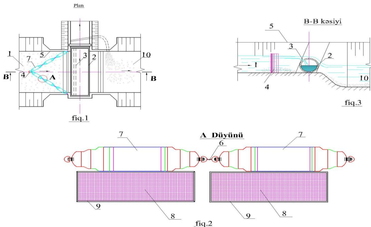
Şəkil 4. Suqəbuledici qurğular üçün balıq mühafizə qurğusunun plan və kəsikləri: yuxarı byef – 1; suqəbuledici qurğu – 2; yarıq – 3; dayaq divar – 4; yan divarlar – 5; oynaq birləşmə – 6; polietilin üzgəc panton – 7; altına kətan və ya geotekstil tor – 8; çürüməyən və paslanmayan metal çərçivə – 9; aşağı byef – 10.
