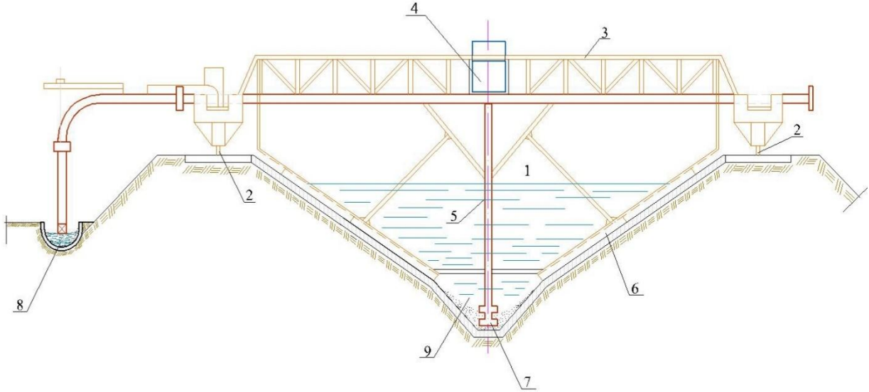
Şəkil 3. Sifonlu durulducu: trapesiya en kəsikli dəmir beton üzlüklü kameranın – 1; oxuna paralel və onun bermaları üzərində qoyulmuş relsdən – 2; metal fermadan – 3; dartıcı mexanizmdən – 4; sifonlu boru – 5; durulducu kamerasının yamacları üzərində qurqşdırılmış sifonlu boruya və metal fermaya bərkidilmiş qaşığıcı bıçaqla – 6; sifonlu borunun ucuna bərkidilmiş sifon – 7; trapesiya en kəsikli dəmir beton üzlüklü kameranın oxuna paralel və kameradan kənarında qoyulmuş yarım silindrik en kəsikli dəmir beton nov – 8; dibi kəsik konus şəkilli dəmir beton üzlüklü xəndək – 9.
