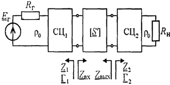
Şəkil1. Bir kaskadlı gücləndiricinin struktur sxemi
