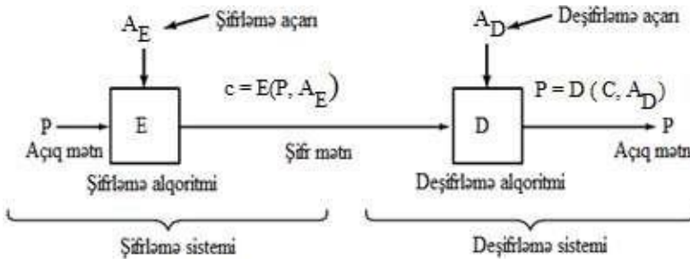
Şək.1.12. Şifrlənmə/deşifrlənmə modeli
