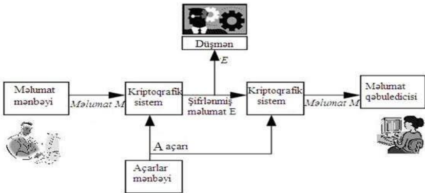
Şək.2.15. Simmetrik şifrləməni istifadə edən məxfi sistemin ümumi strukturası
