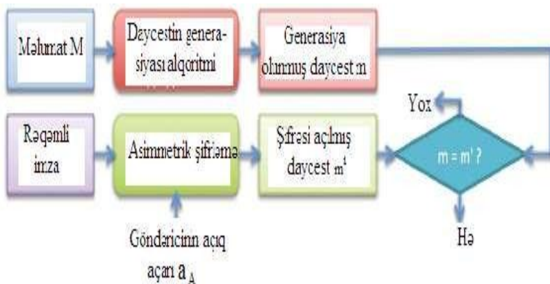
Şək.3.8. Elektron rəqəmli imzanın yoxlanılması sxemi
