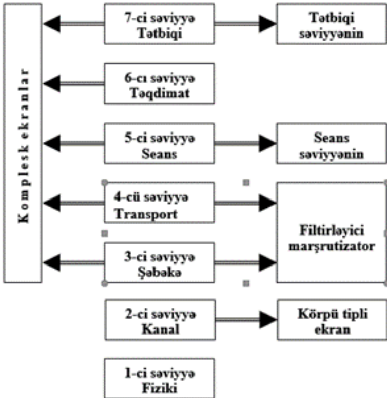
Şək.1.2. Şəbəkəlararası ekranın Open Systems Interconnection modelinin fərqli səviyyələrində həyata keçirilməsi
