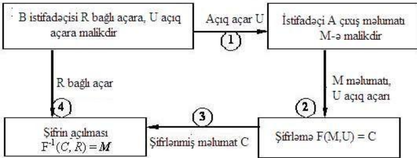
Şəkil 3.1. Açıq şifrələmə sxemi
