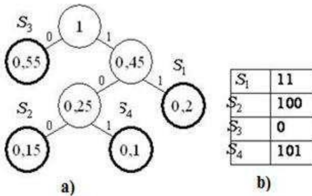
Şək.4.3. Xofman kodlamasının ikinci mərhələsi ayrı qovşaqlarını birləşdirən qabırqalar 0 və 1 rəqəmləri ilə nömrə-lənirlər (məsələn, sol qabırqa-“0”-la, sağ qabırqa isə 1-lə).
