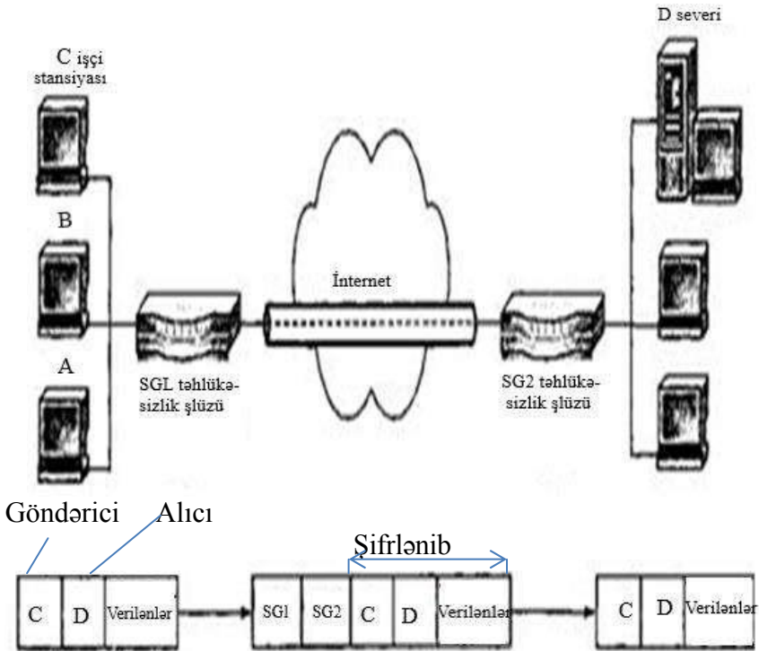
Şəkl. 5.3. Bərpa olunmuş başlıqlı paketin alınması və onun şəbəkə üzrə ötürülməsi sxemi
