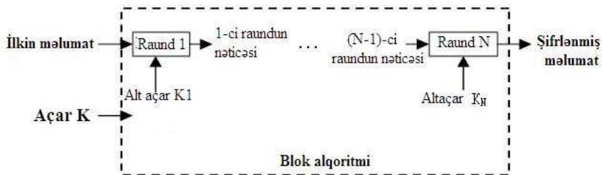
Şək. 2.6. Simmetrik şifrələmənin blok alqoritminin strukturu
