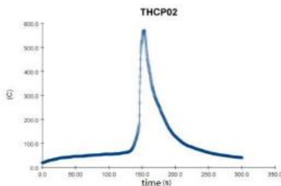
Şəkil 3. Yanğıın mənbəyinin yaxınlığında temperatur qeydi nöqtəsi
