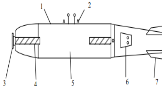
Şəkil 1. Hava bombasının eskiz xəritəsi 1-qabıq gövdəsi, 2-qaldırıcı qapaq, 3-funq, 4-gücləndirici taxıl, 5-əsas yük, 6-qapaq, 7-empennaj
