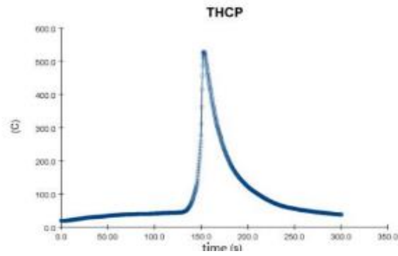
Şəkil 4. Uzaq yangın mənbəyinin temperatur qeyd nöqtəsi
