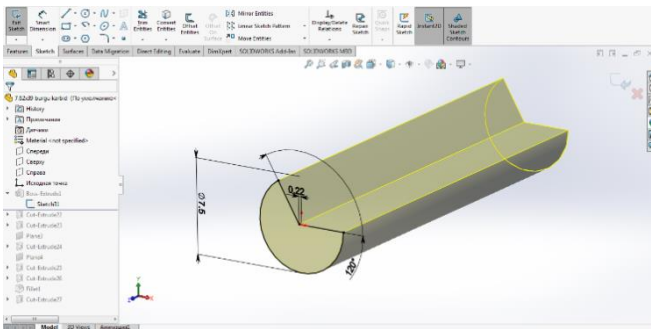
Şəkil 1. Burğunun kəsici hissəsinin modelləşdirilməsi
