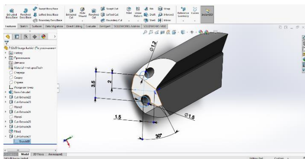
Şəkil 5. Burğuda soyuducu-yağlayıcı mayenin kontakt sahəyə çatdırılması üçün kanalın açılması
