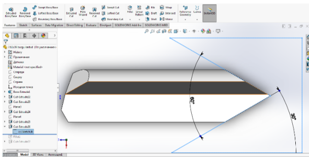
Şəkil 4. Burğunun kəsici və gövdə hissələrinin birləşmə zonasının modelləşdirilməsi
