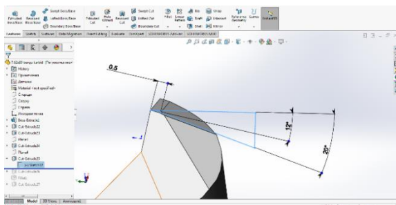
Şəkil 3. Burğunun əsas kəsici tilinin modelləşdirilməsi
