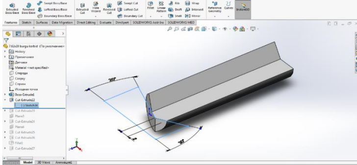
Şəkil 2. Burğunun qabaq və arxa üzlərinin modelləşdirilməsi
