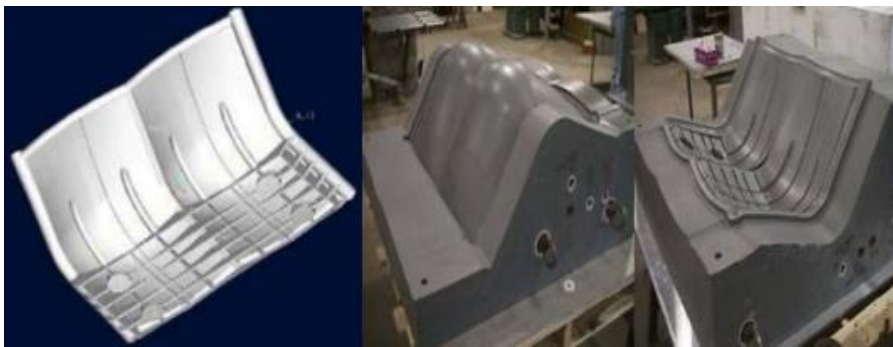
Şəkil 3. Kompozit Oturacaq Dizaynı və Qəlibləri
