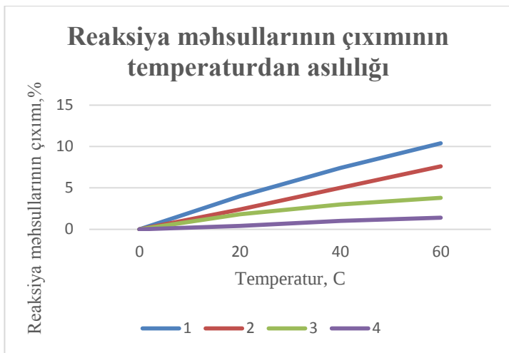
Şəkil 2. Reaksiya məhsullarının çıxımının temperaturdan asılılığı: V_{\text{CH}_4}=0,086 l/saat, V_{\text{H}_2\text{O}_2}=0,8 ml/saat, C_{\text{H}_2\text{O}_2}=20\% , \text{CH}_4:\text{H}_2\text{O}_2=1:1,4 (mol) 1- \text{CH}_4 konversiyası, 2-metanol, 3 və 4 - \text{CH}_2\text{O} və \text{HCOOH} , 4-selektivlik.
