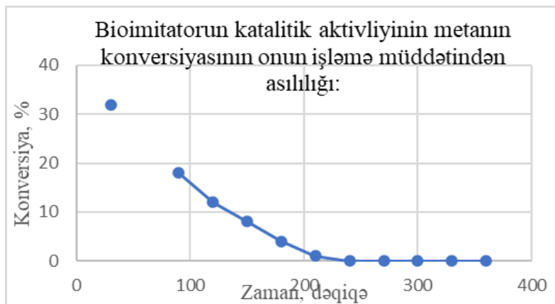
Şəkil 1. Bioimitatorun katalitik aktivliyinin metanın konversiyasının onun işləmə müddətindən asılılığı: t=180^{\circ}\text{C} , T=13 sek, V_{\text{CH}_4}=0,086 l/saat, V_{\text{H}_2\text{O}_2}=0,8 ml/saat, \text{CH}_4:\text{H}_2\text{O}_2=1:1,4 (mol), C_{\text{H}_2\text{O}_2}=20\%
