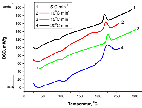
Şəkil 1. XŞY Se 95 Te 5 tərkibinin 5, 10, 15 və 20 K/dəq qızdırılma sürətlərində DSK əyriyələri.
