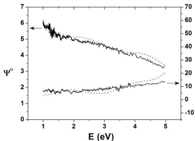
Рисунок 4. Параметры спектроскопической эллипсометрии для нанокompозита с концентрацией наночастиц \text{Bi}_2\text{Te}_3 30%. Сплошной линией обозначены экспериментальные данные, штриховой линией обозначены расчётные данные.
