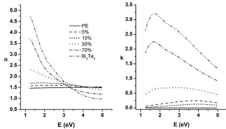
Рисунок 3. Показатели преломления и экстинкции, рассчитанные при указанных номинальных концентрациях, в диапазоне энергий 1-5 eV.
