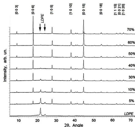
Рисунок 1. Дифракция рентгеновских лучей в нанокомпозитах LDPE - \text{Bi}_2\text{Te}_3 с различной концентрацией наночастиц (5%, 10%, 30%, 40%, 50%, 60% и 70%).
