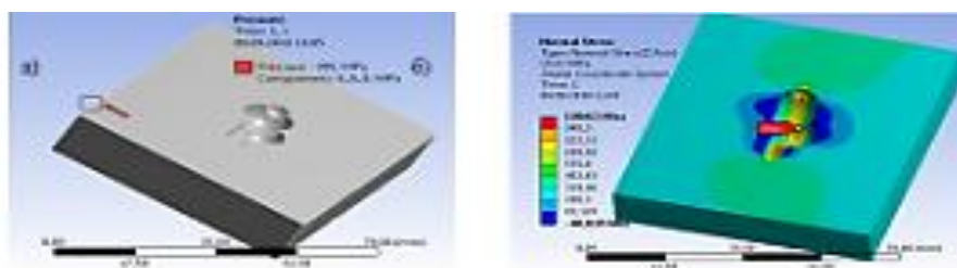
Şəkil 3. Korroziya qüsuru olan hesablama modeli: a) yüklər və sərhəd şərtləri; b) qüsurlu hissəsində gərginliklərin hesablanması nəticələri
