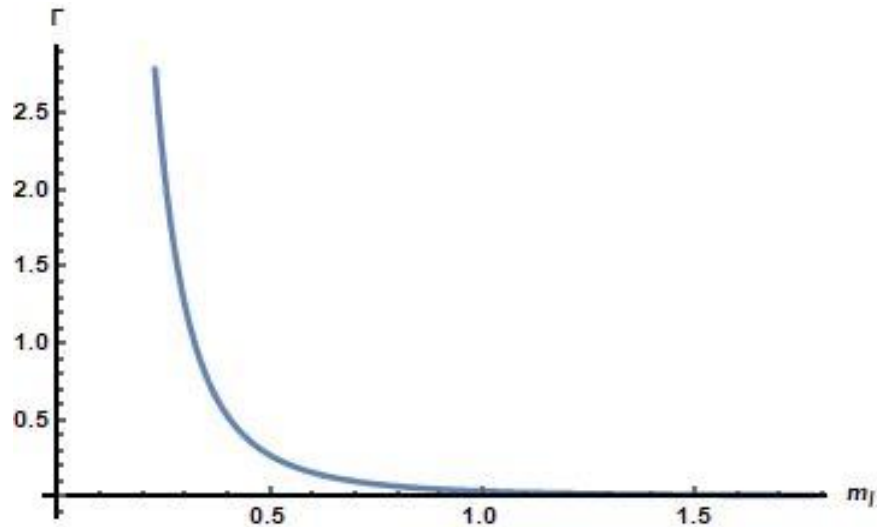
Рис. 4. Зависимость ширины распада процесса H \rightarrow Z^*Z^* \rightarrow 4l от массы лептона m_l .
