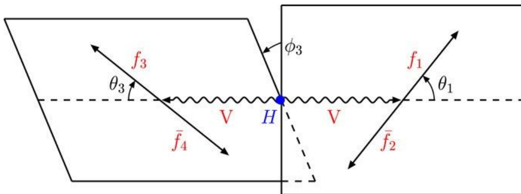
Рис. 2. Определение полярных и азимутальных углов.
