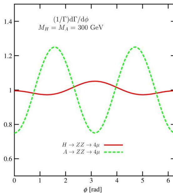
Рис. 3.2.3. Распределение ширины распада H \rightarrow Z^*Z^* \rightarrow 4\mu по азимутальному углу.
