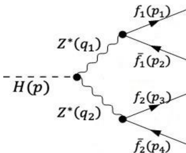
Рис. 1. Фейнменовская диаграмма процесса H \rightarrow Z^*Z^* \rightarrow 4l .
